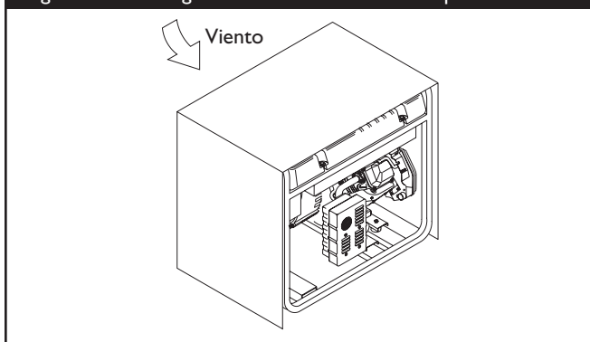
Figura 19 — Refugio Frío Permanente del Tiempo
